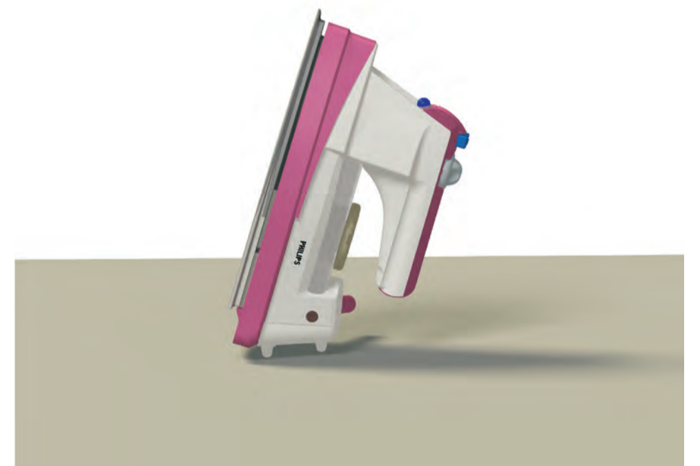
Renders da modelação do re-design do ferro de engomar obtidos a partir do SolidWorks.
