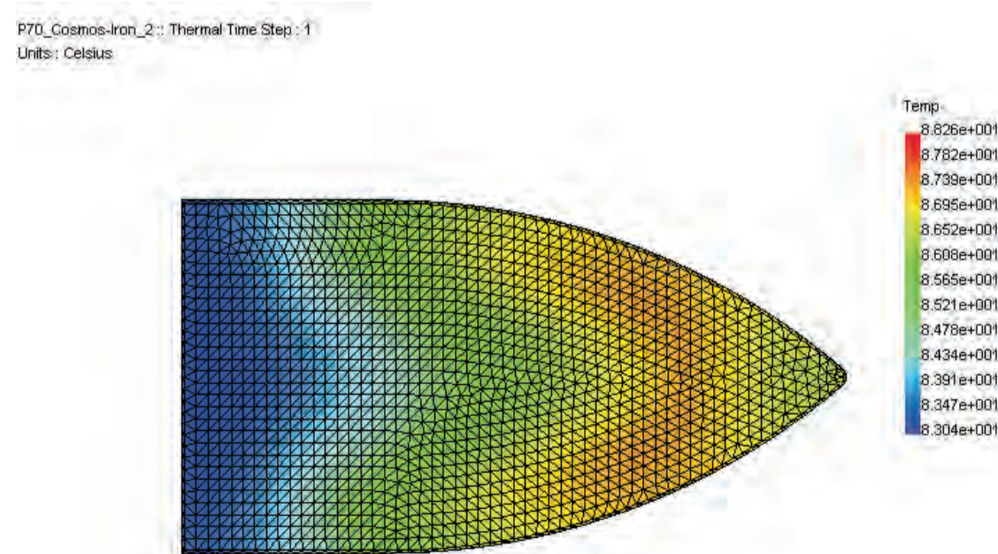
Análise térmica através do método de elementos finitos obtido a partir do CosmosWorks.
